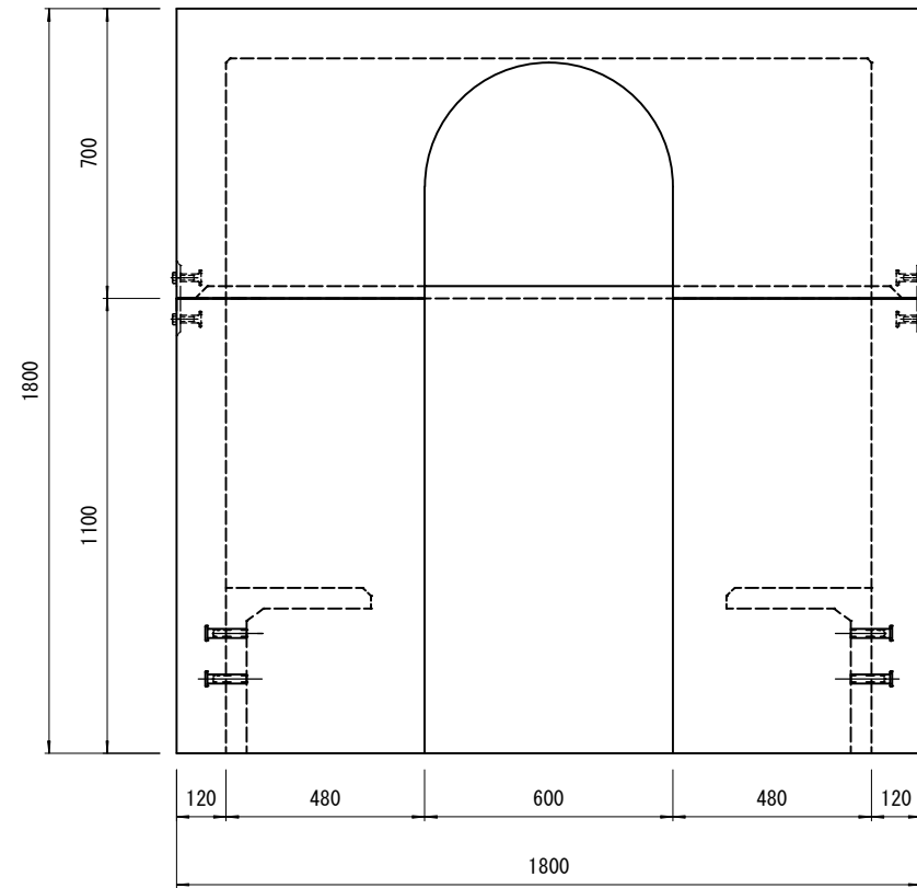
正面図
