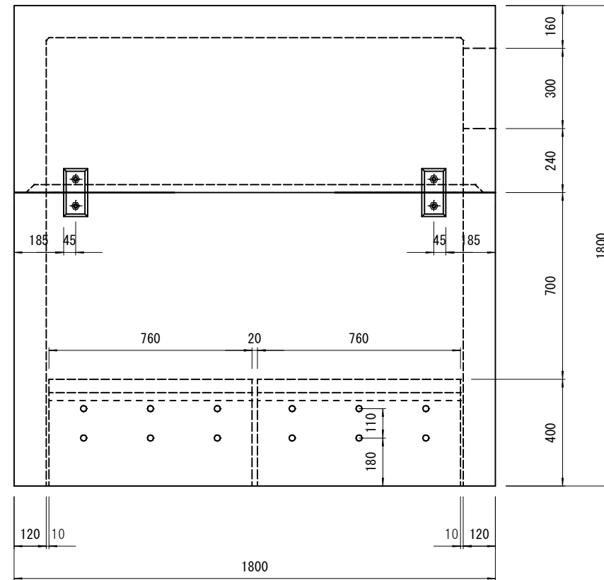
側面図
